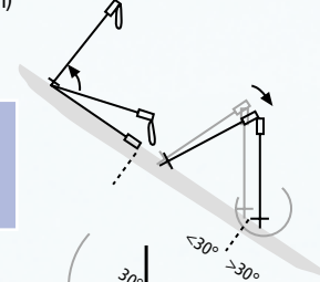
Mesure de la déclivité à l'aide de bâtons: triangle équilatéral, méthode du pendule.
